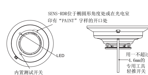
图4、内置测试开关位置及SENS-RDR位置示意图：
