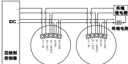
图3、布线图：
