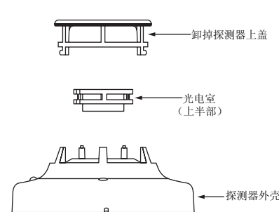
图5、探测器拆卸/安装示意图：
