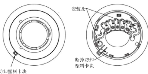
图2、防卸功能示意图：
